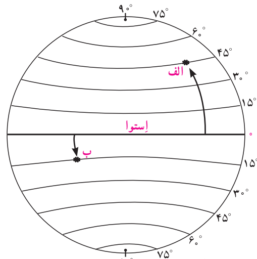
عرض جغرافیایی الف — 45^{\circ}N (۴۵ درجه شمالی) ب — 15^{\circ}S (۱۵ درجه جنوبی)
